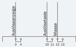
Anschlussbelegung RWA-Taster 7
