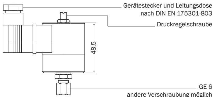
Pneumatisch-Elektrischer Druckschalter (Signalwandler)
